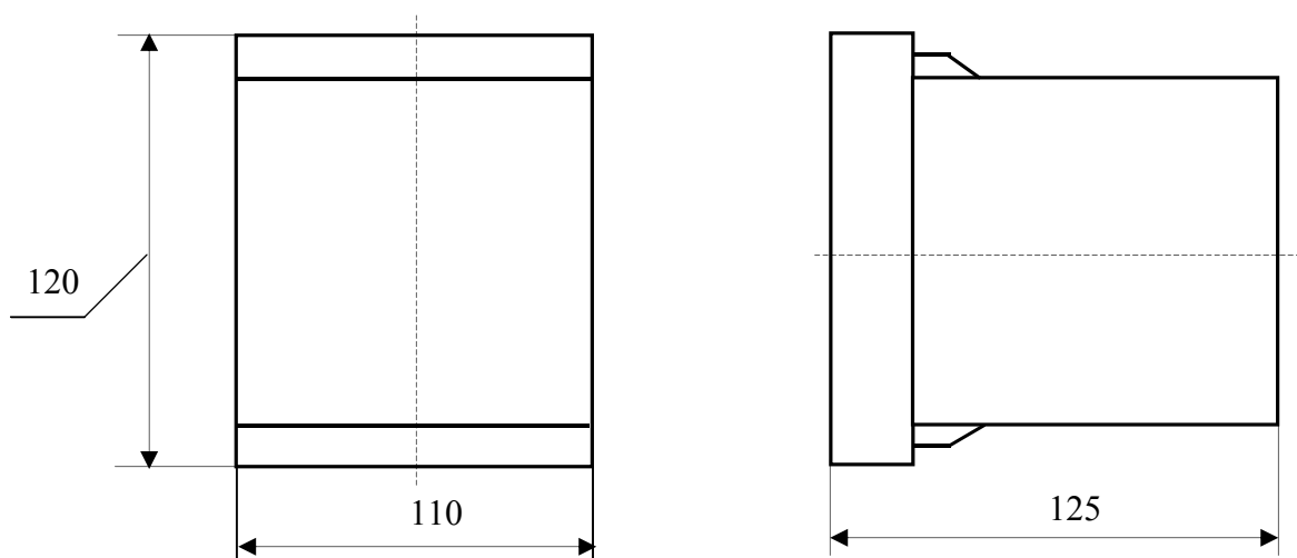
Рисунок А.1 – Габаритные размеры ИП
